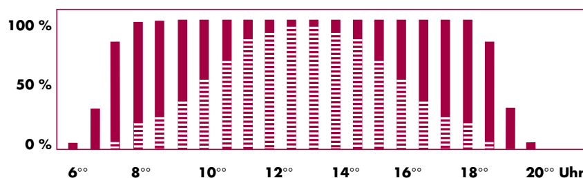
Leistungsdiagramm am Beispiel eines sonnigen Sommertages starr DEGERtraker
